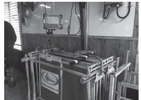
Tru-Test XR5000 + bâton RFID Syscan + cellules de pesée
